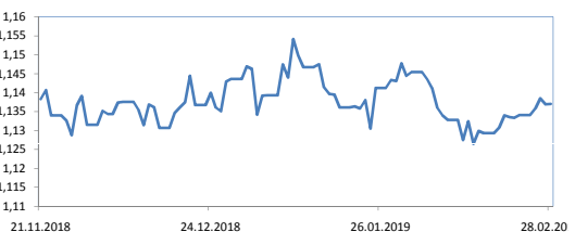
Динамика CDS
