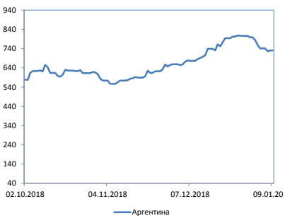
Динамика CDS
