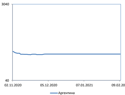
Динамика CDS
