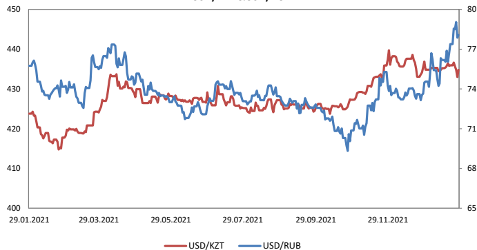
USD/KZT & USD/RUB
